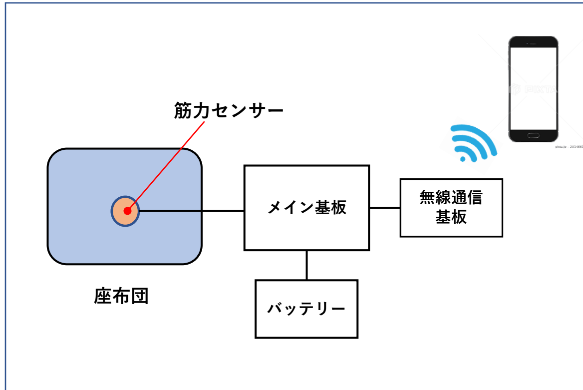
実験機のシステム構成
