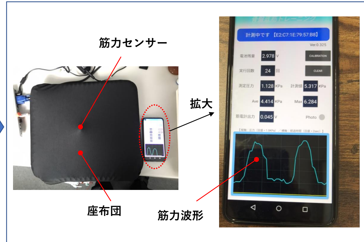
実験機による筋力計測の写真
